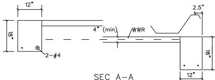
SEC A-A
