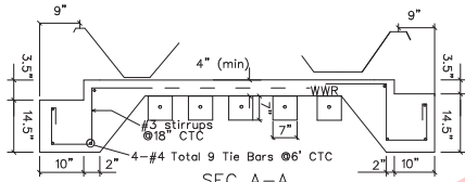
SEC A-A
